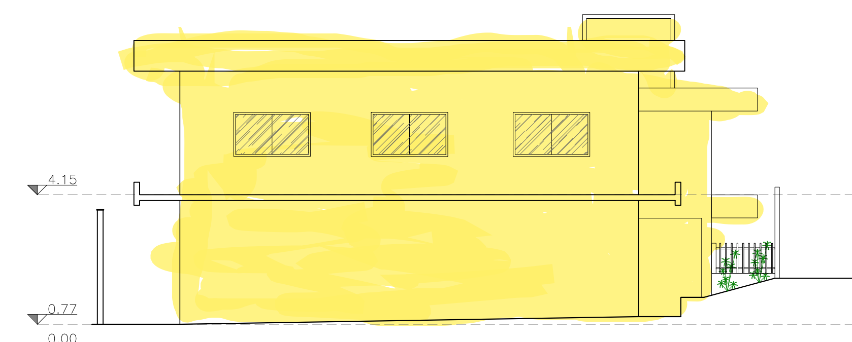
ELEVAÇÃO 04
