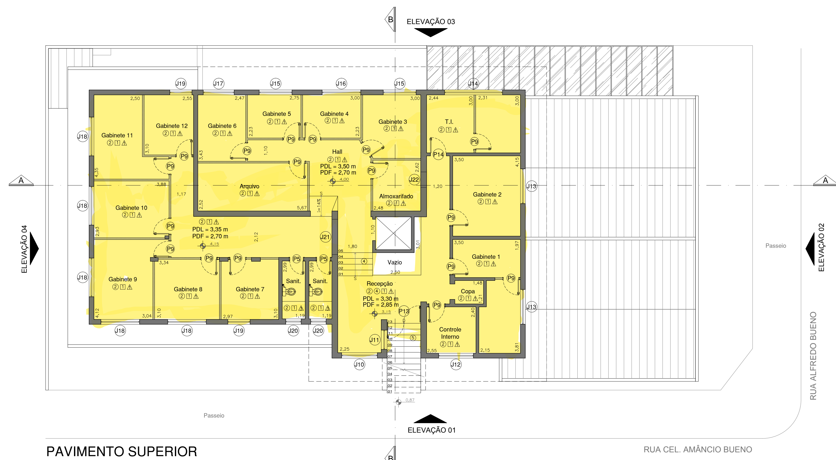
PAVIMENTO SUPERIOR
