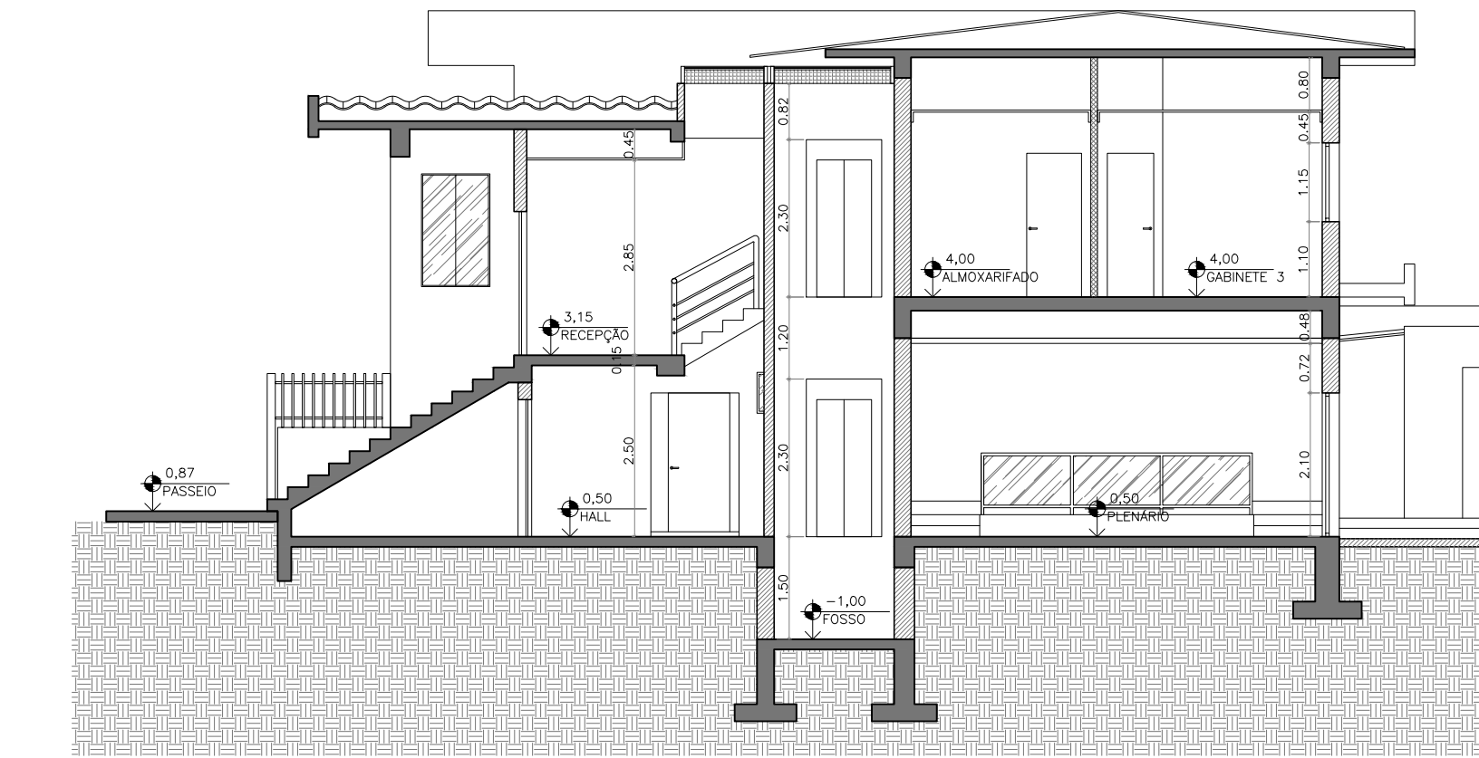
CORTE BB
